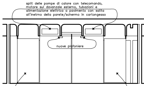
SEZIONE A-A
